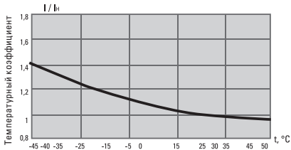
Рисунок 4. Температурный коэффициент для АД-32
